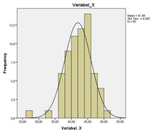
Gambar 4.1 Histogram Distribusi Frekuensi Variabel X
